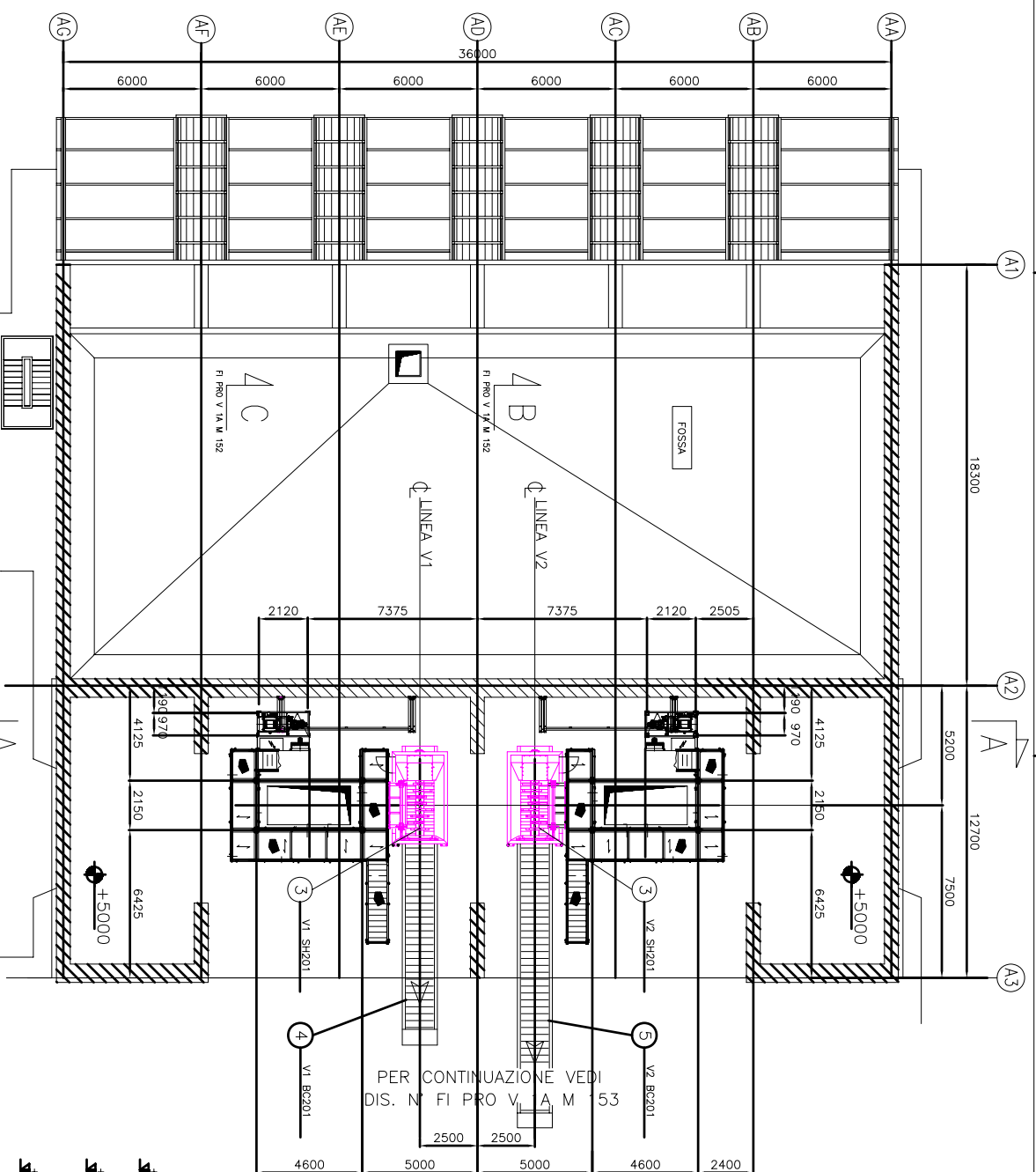
PIANTA A +5000
